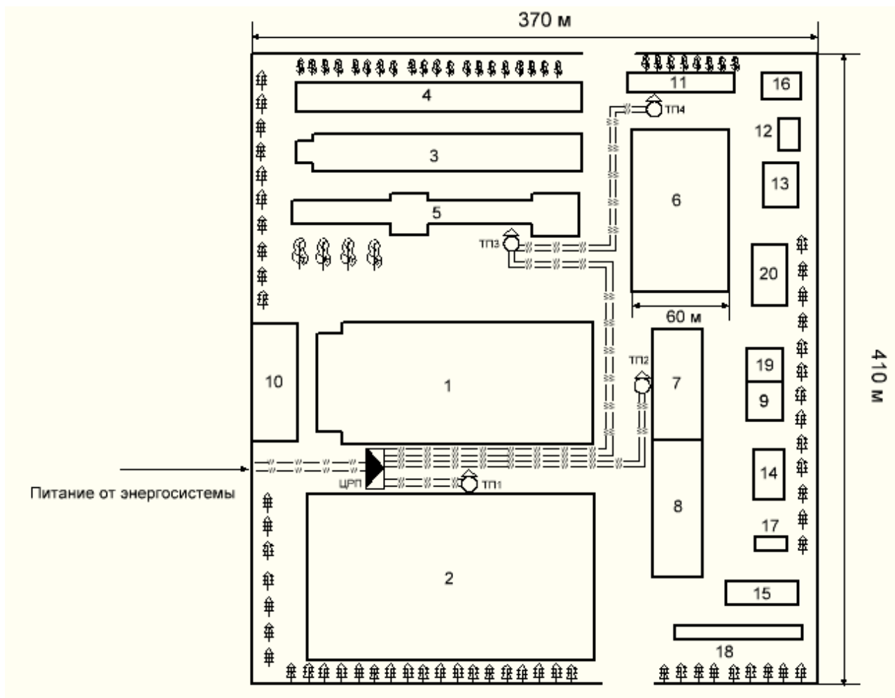
Рисунок 1.1 - Генеральный план проектируемого предприятия
