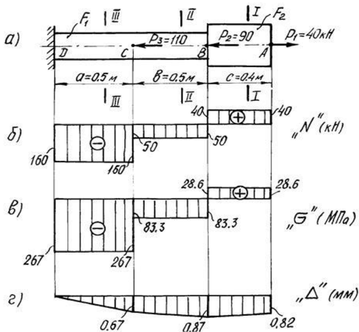
Рис. 2. Расчетная схема бруса и эпюры: а - расчетная схема; б - эпюра продольных сил; в - эпюра напряжений; г - эпюра продольных перемещений
