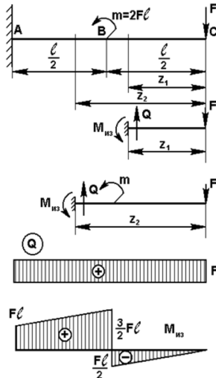
Рис.1а. Расчетная схема
