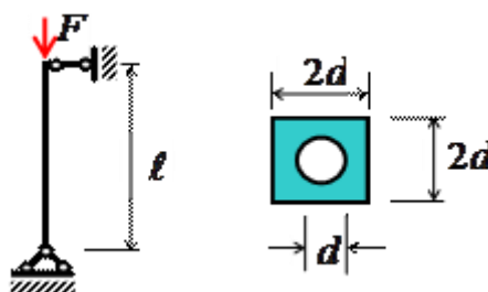
Рис. 17. Расчетная схема
