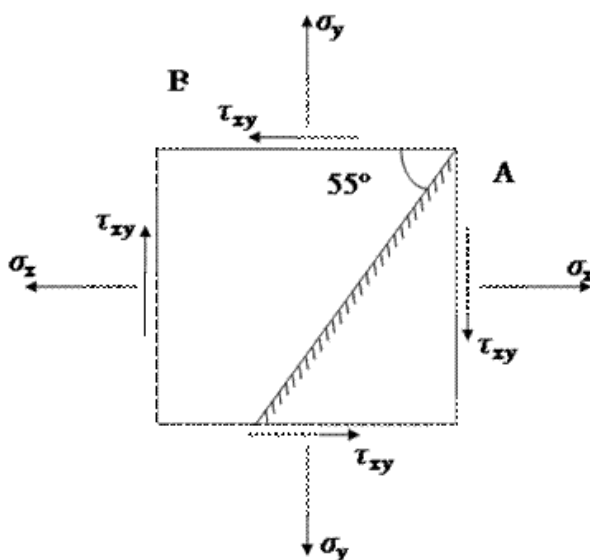
Рис.4. Расчетная схема
