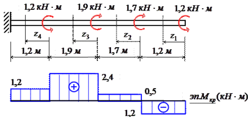
Рис. 9. Расчетная схема
