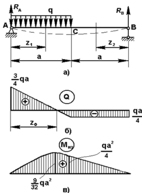
Рис.1в. Расчетная схема
