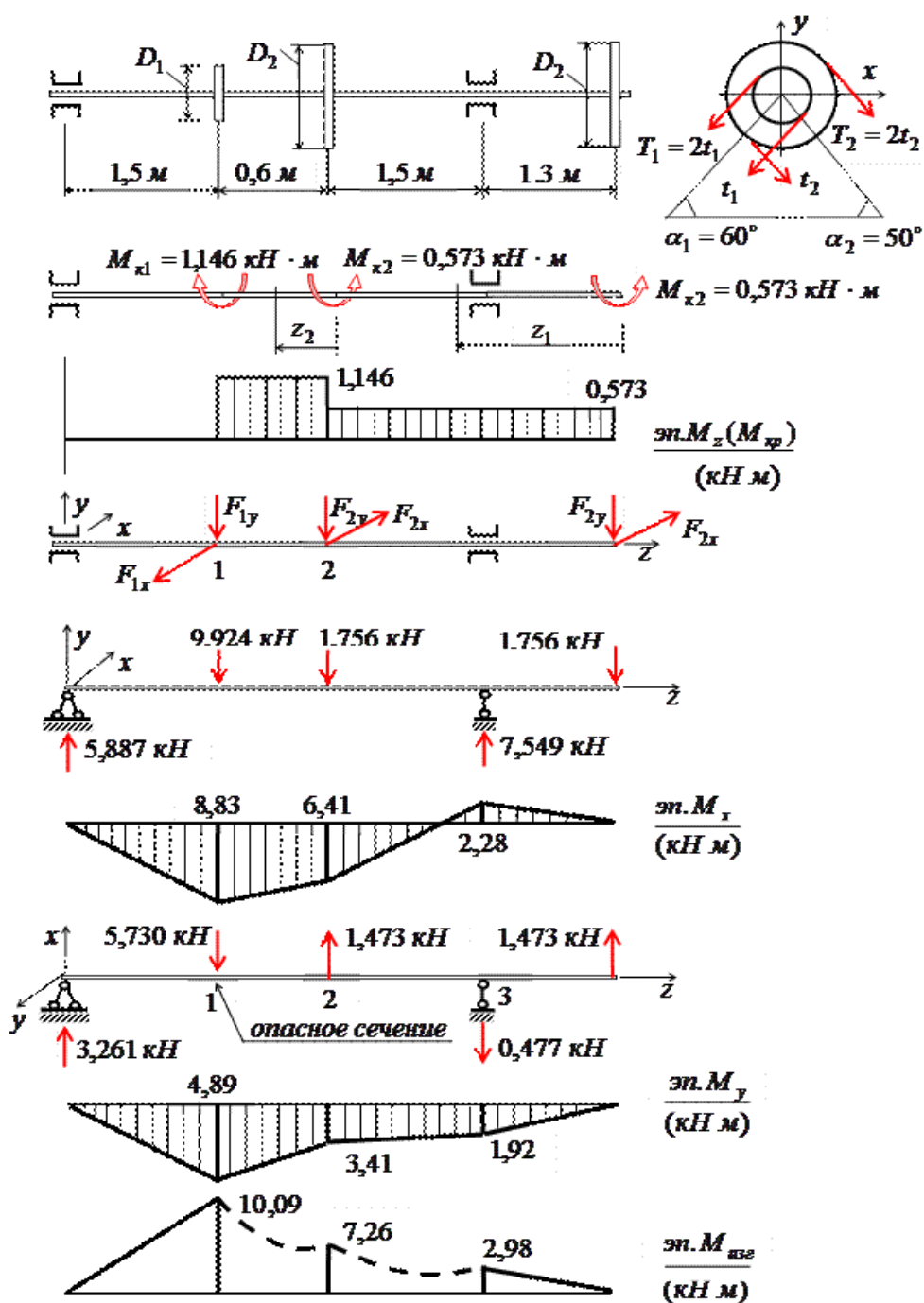
Рис. 16. Расчет вала
