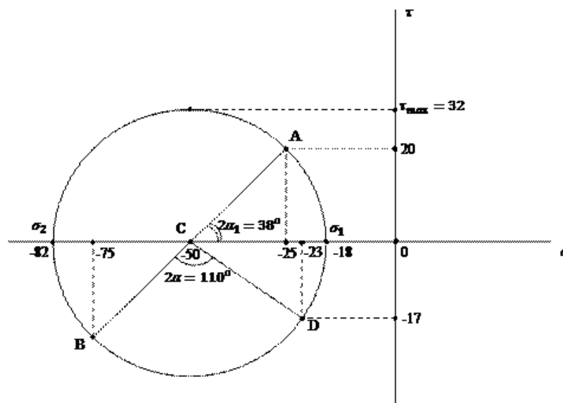
Рис. 5. Круг Мора
