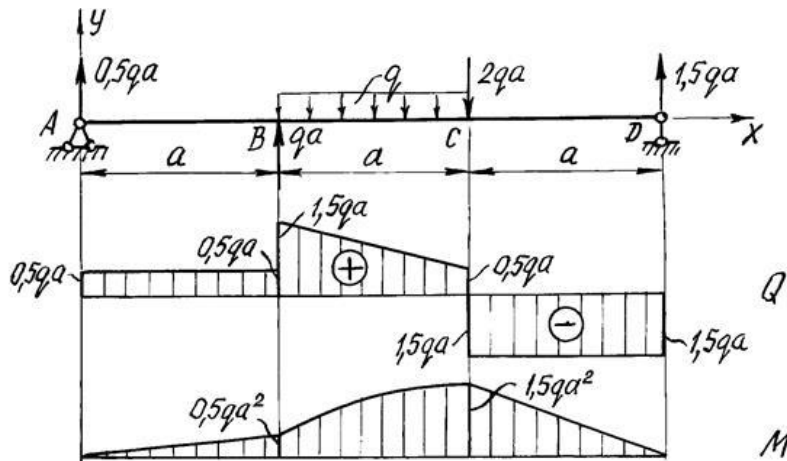
Рис. 11. Эпюры поперечных сил и изгибающих моментов
