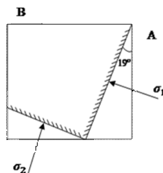
Рис.6. Положение главных площадок и направление главных напряжений
