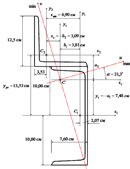
Рис. 9. Расчетная схема
