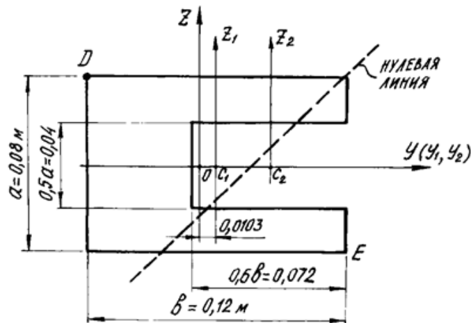
Рис. 13. Поперечное сечение бруса
