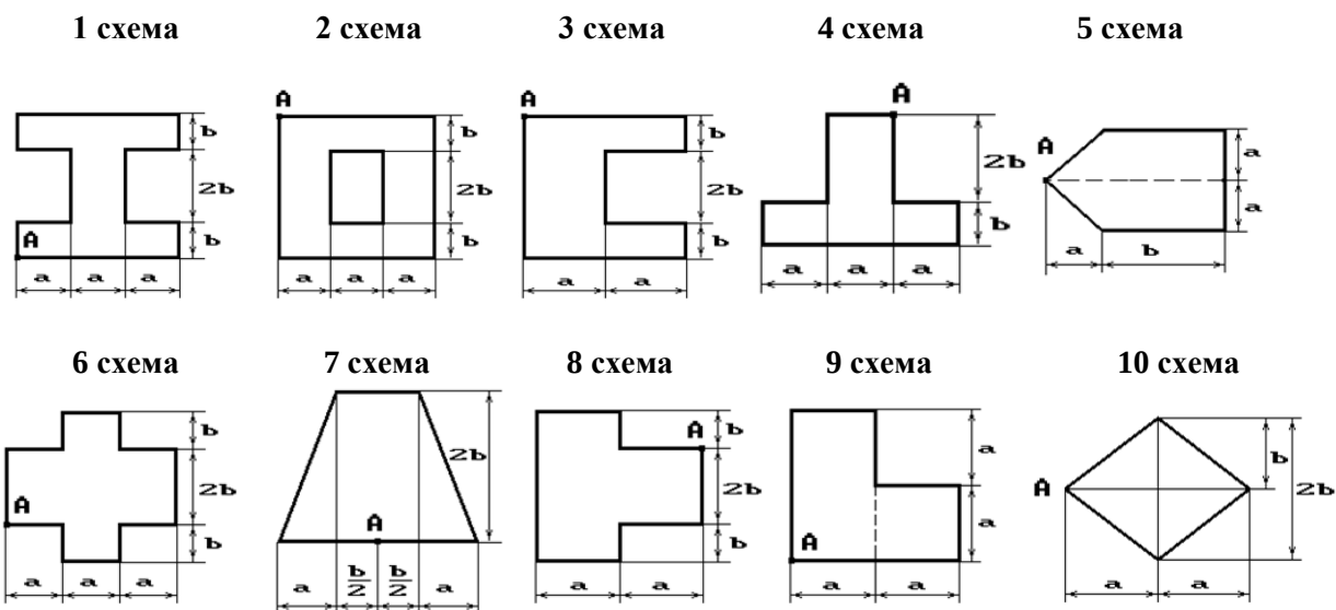
Рис.12. Поперечное сечение
