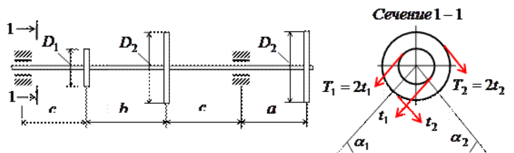
Рис. 15. Расчетная схема
