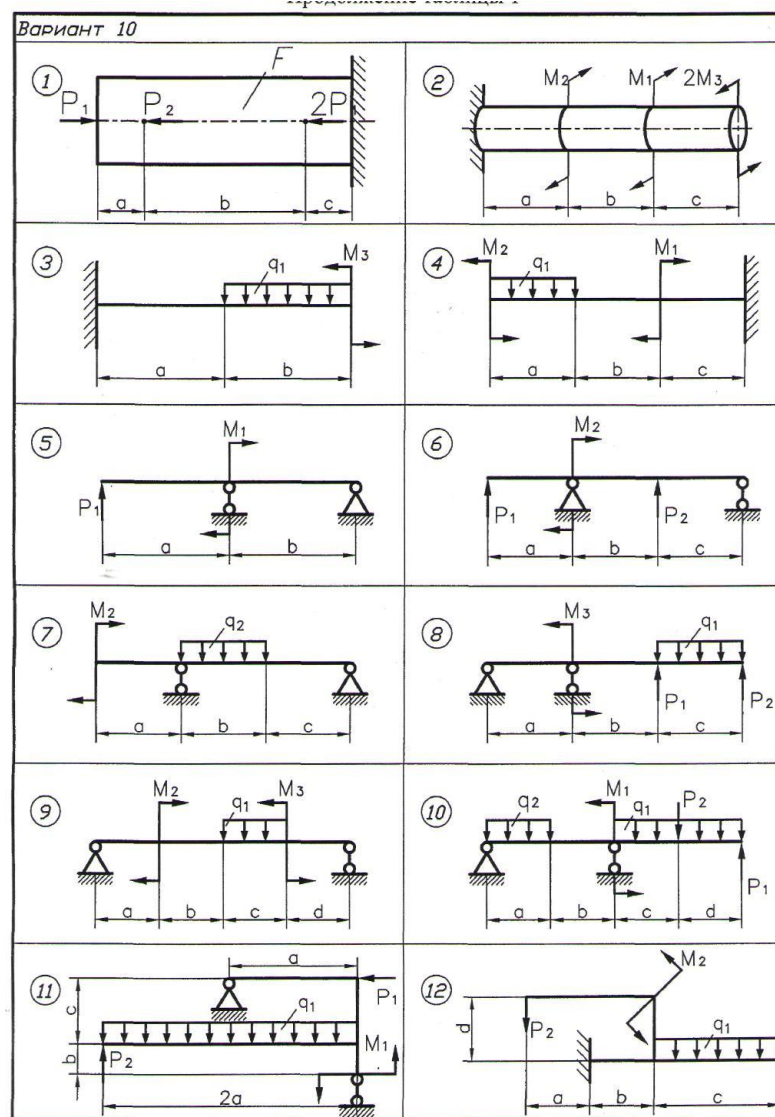
Рис.1. Расчетные схемы
