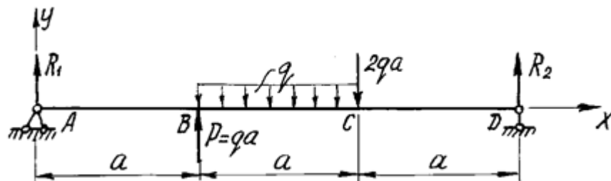
Рис. 10. Расчетная схема балки
