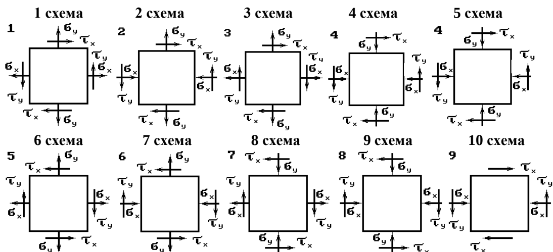
Рис. 3. Расчетные схемы
