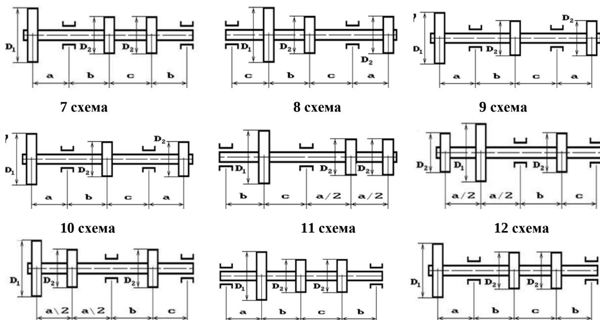
Рис. 14 Расчетные схемы
