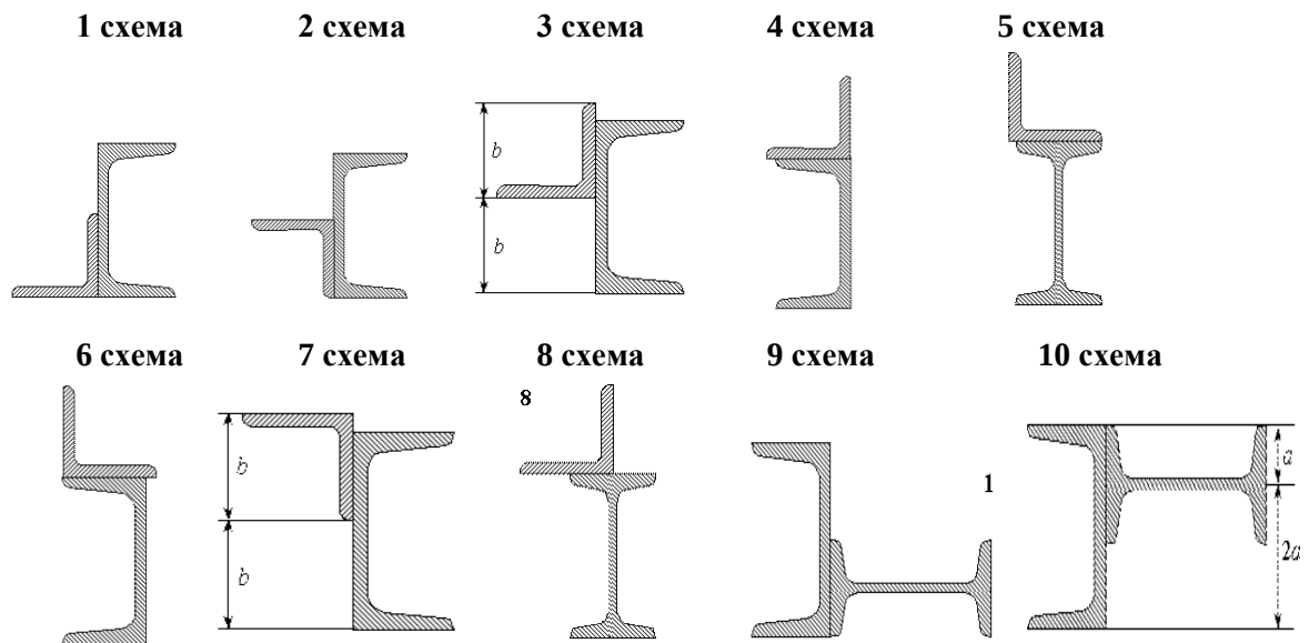
Рис. 7. Расчетные схемы
