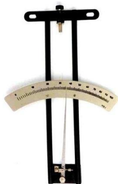
Рисунок 2– Гигрометр.
