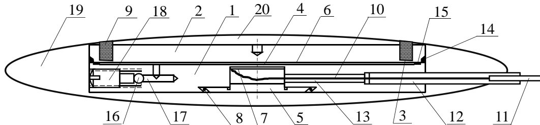
Рис. 2. Конструкция месдозы в эллипсоидном корпусе в сборе 1 – корпус месдозы, 2 – приемный диск, 3 – кольцевая мембрана, 4 – измерительная мембрана, 5 – массивная крышка, 6 – полость для силиконовой жидкости, 7 – тензорезистор, 8 – запорное кольцо, 9 – резиновое кольцо, 10 – провод, 11 – кабель, 12 – вкладыш, 13 – эпоксидная смола, 14 – место для пайки, 15 – прокладка из клея, 16 – запорный шарик, 17 – канал для заполнения силиконовой жидкостью, 18 – специальный винт, 19 – эллипсоидный пластмассовый корпус, 20 – пластмассовая накладка над приемным диском.
