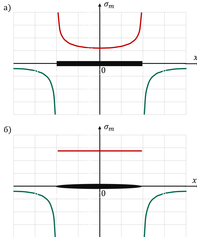
Рис. 1. Характерные графики распределения нормального давления: а – для месдозы в виде цилиндрического диска, б – для месдозы в виде эллипсоидного диска
