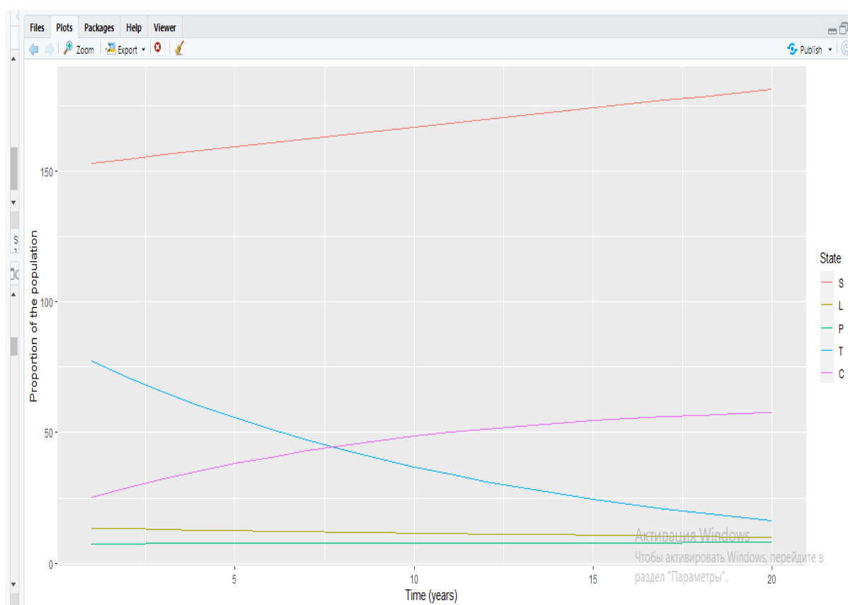
Рис.1. График модели на языке R
