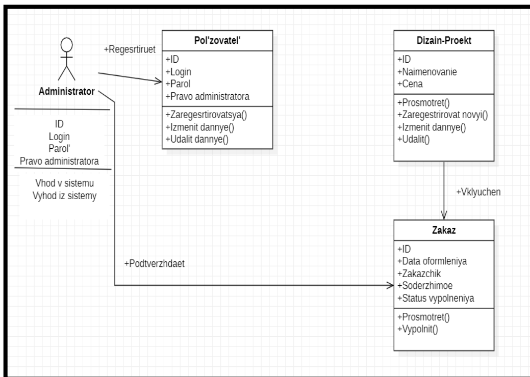
Рисунок 3 – Диаграмма классов.
