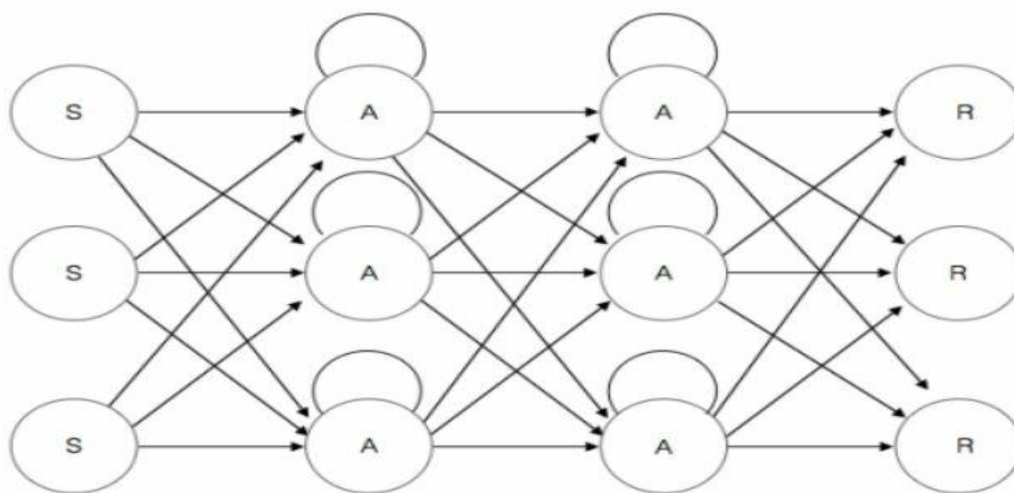
Рис.2. Схема RNN.
