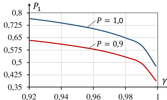
Рис. 2. Зависимость нижнего предела доверительного интервала P_1 от вероятности заданной надежности \gamma .
