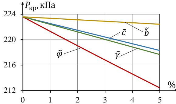
Рис. 1. Влияние изменчивости \tilde{\varphi} , \tilde{c} , \tilde{\gamma} и \tilde{b} на величину критической нагрузки
