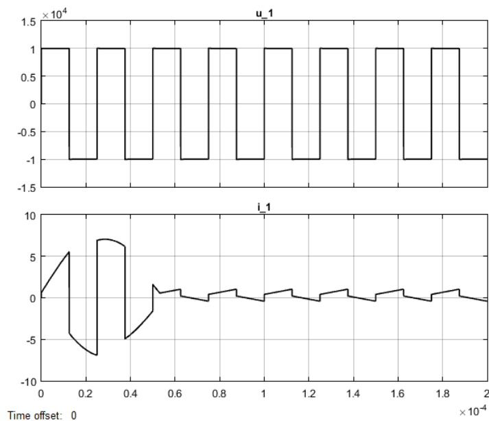
Рис. 6 Кривые напряжения и тока на начальном этапе при включении трансформатора на холостом ходу
