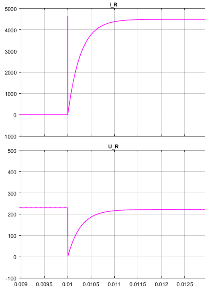
Рис. 8 Ток и напряжение на сопротивлении нагрузки
