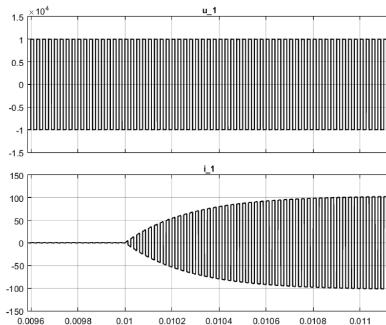
Рис. 5. Напряжение и ток инвертора при набросе номинальной нагрузки
