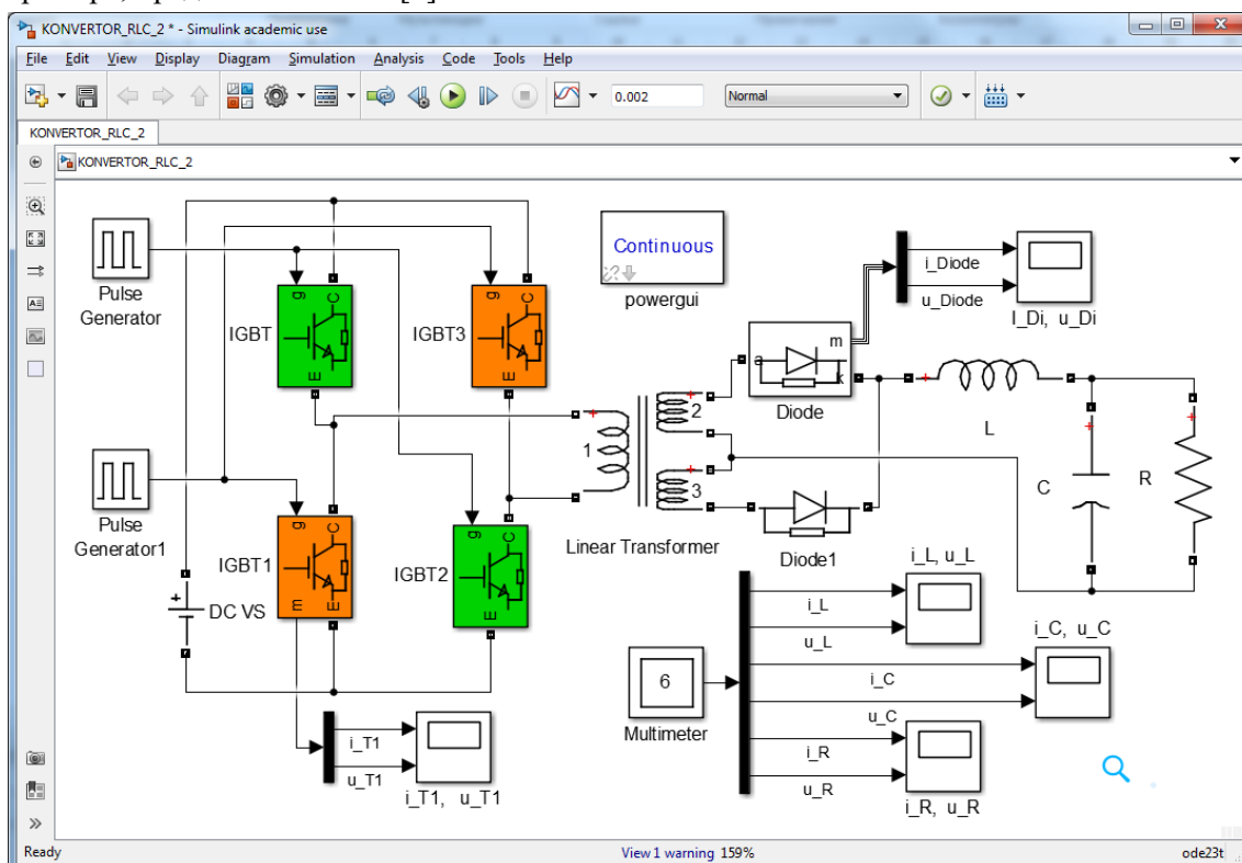
Рис. 1 Модель силового полупроводникового трансформатора постоянного тока
