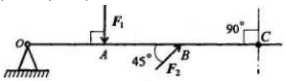
Плоская система произвольно расположенных сил
