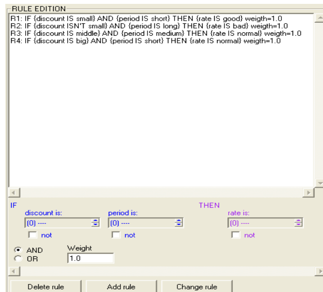
Рис.2.7. Редактор правил вывода
