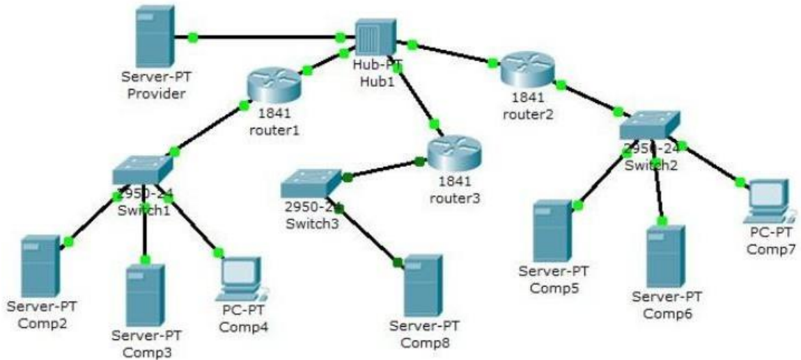
Рисунок 1. Схема сети
