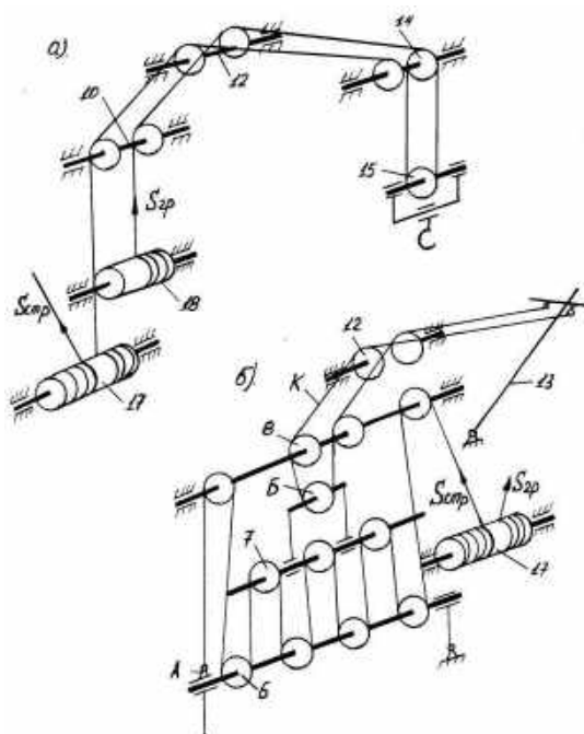
Рисунок 5.2 - Схемы запасовки канатов грузового «а» и стрелового «б» полиспастов
