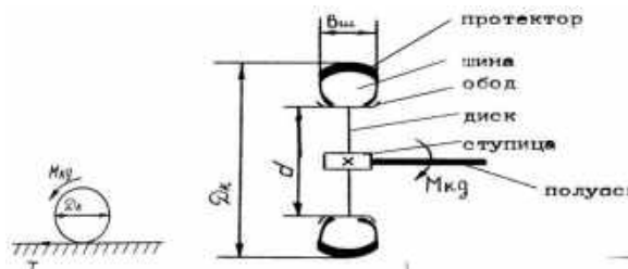
Рисунок 2.3 - Устройство колесного движителя автомобиля
