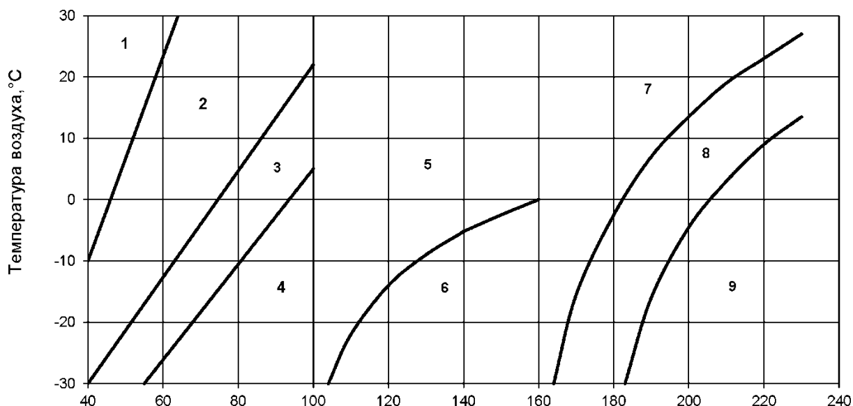
Рисунок 3 - Номограмма для эксплуатационной оценки бензинов:
