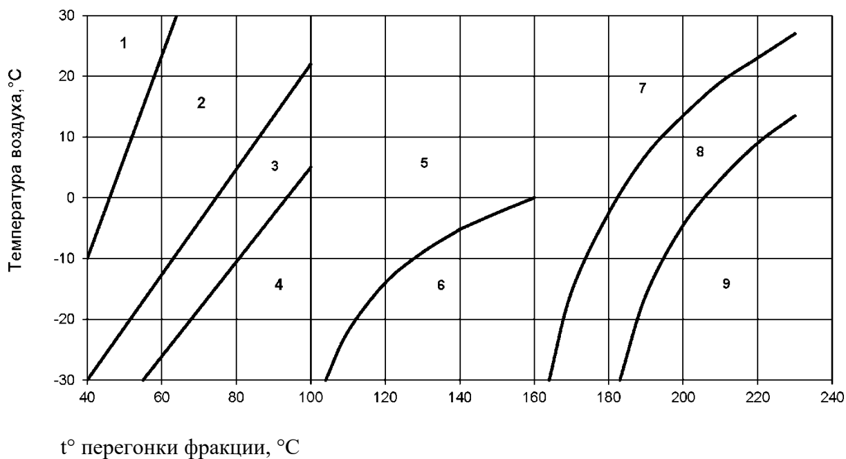
Рисунок 3 - Номограмма для эксплуатационной оценки бензинов:
