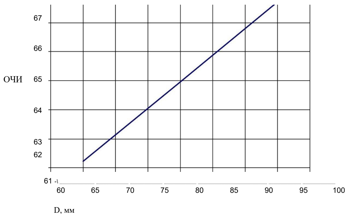
Рисунок 1 - Зависимость требуемого октанового числа бензина при различных значениях диаметра цилиндра при степени сжатия \epsilon равной 5,5 единиц
