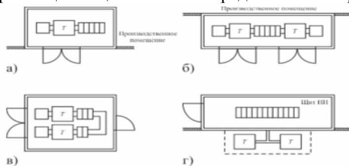
Рис.6. 1 – Варианты размещения цеховых КТП и их компоновки: а – однитрансформаторная КТП встроенного типа; б – двухтрансформаторная КТП пристроенного типа однорядного исполнения; в – двухтрансформаторная КТП отдельно стоящая двухрядного исполнения; г – КТП с наружной установкой трансформаторов
