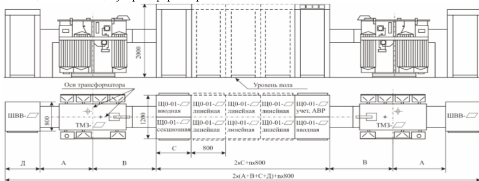
Рис. 1. План двухтрансформаторной КТП однорядного расположения со стационарными выключателями
