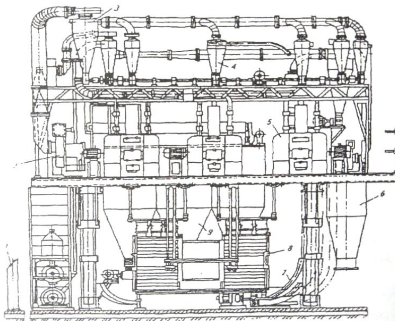
Рис. 2 – Агрегатная вальцовая мельница АВМ-ЗМ
