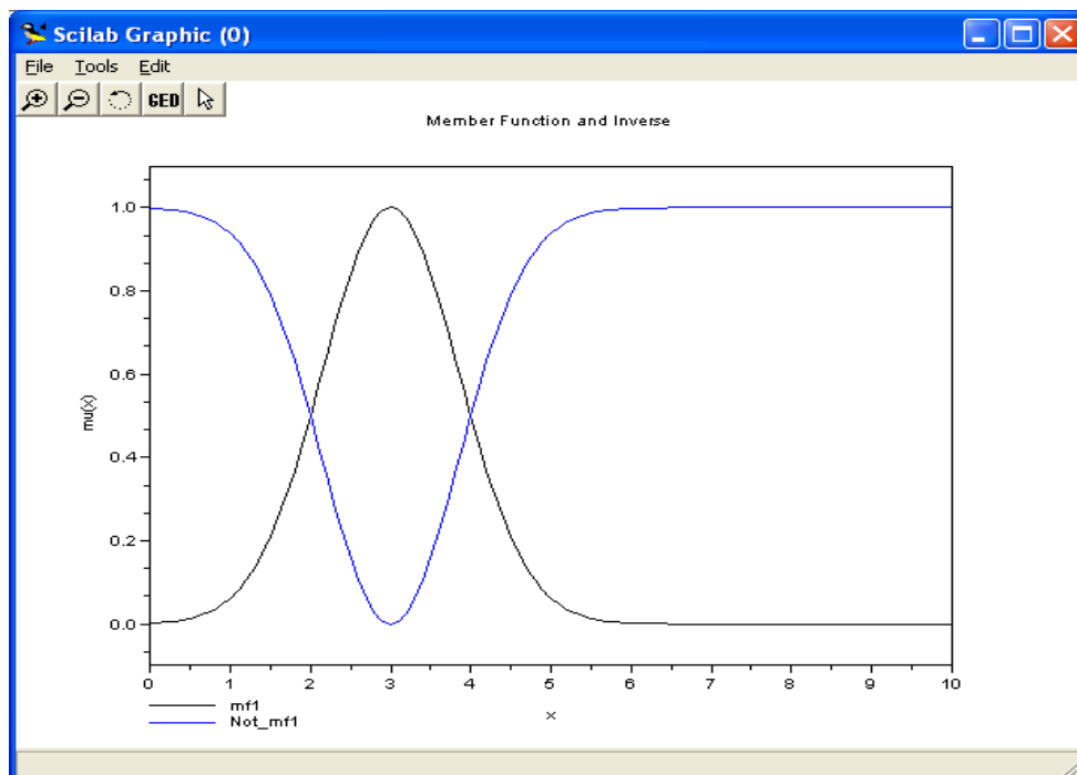
Рис.1.8. Функция дополнения
